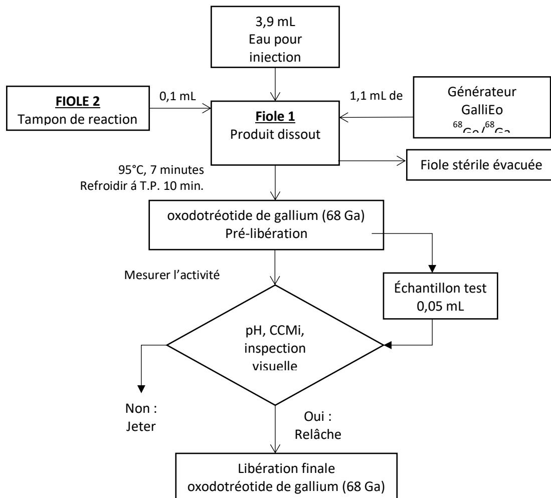
Figure 1 : Procédure de reconstitution pour le générateur Galli Eo d'IRE
