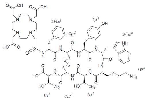
Figure 2 Structure chimique de l'oxodotrétotide
